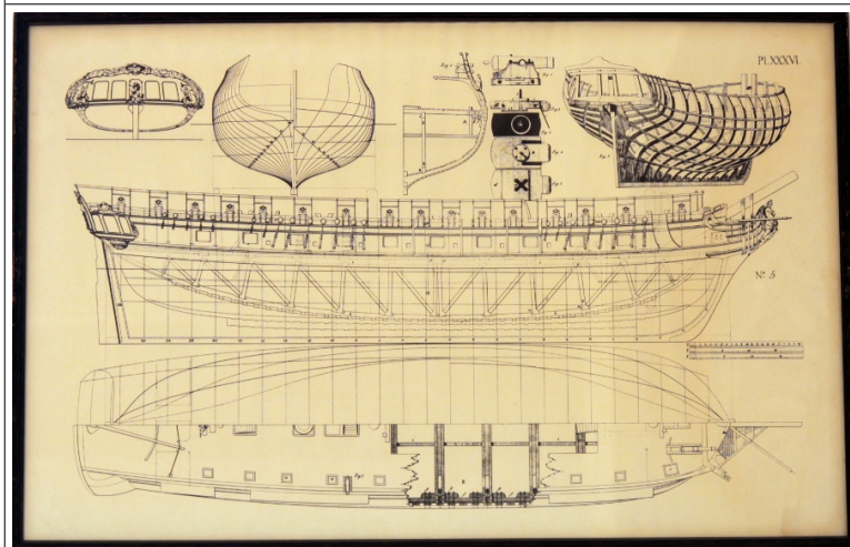
Fartygsritning. Tryck. 41 x 63 cm. 200 kr.
